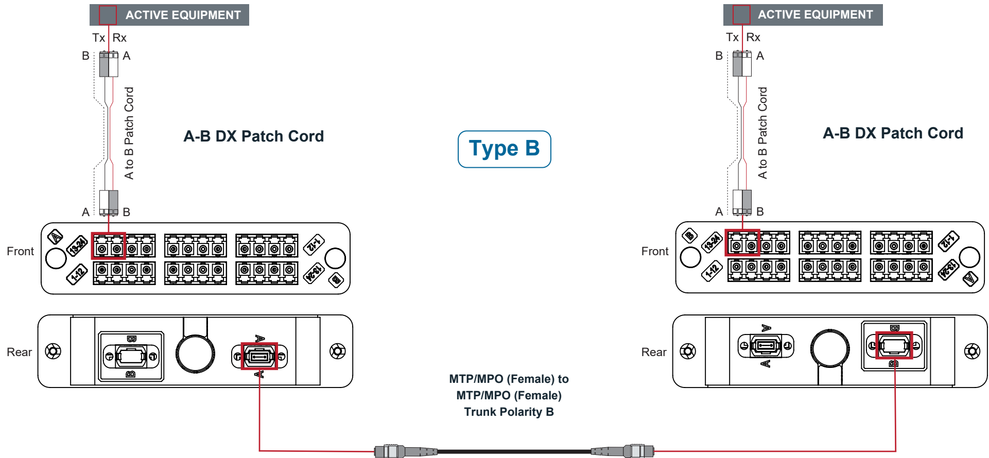
Type B Universal MTP/MPO - LC Module
