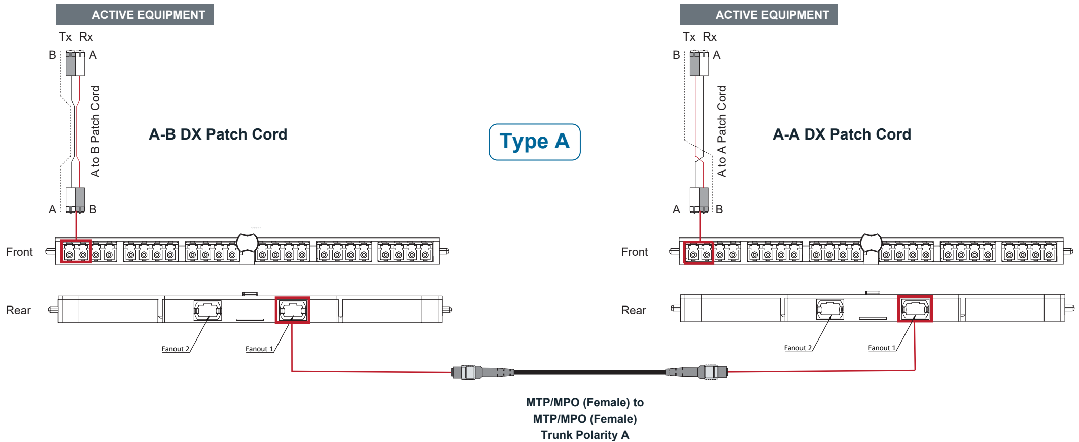
Type A/C MTP/MPO - LC Module
