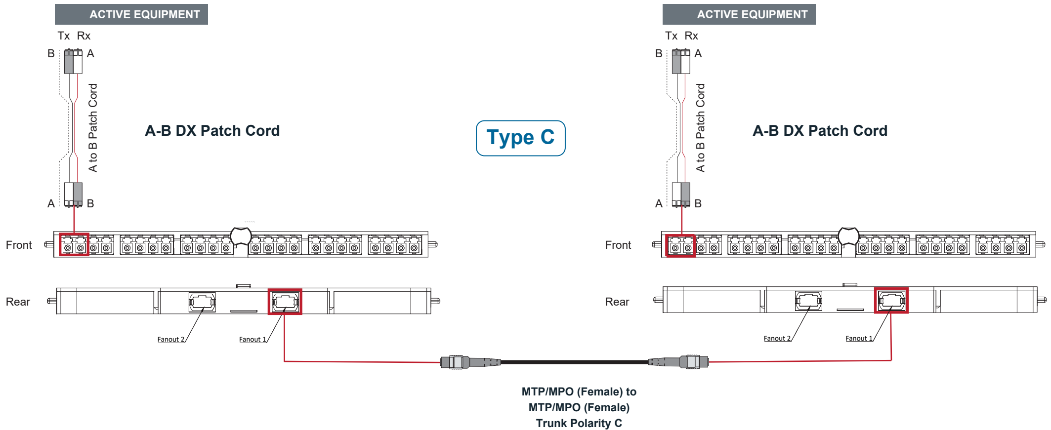
Type C MTP/MPO - LC Module
